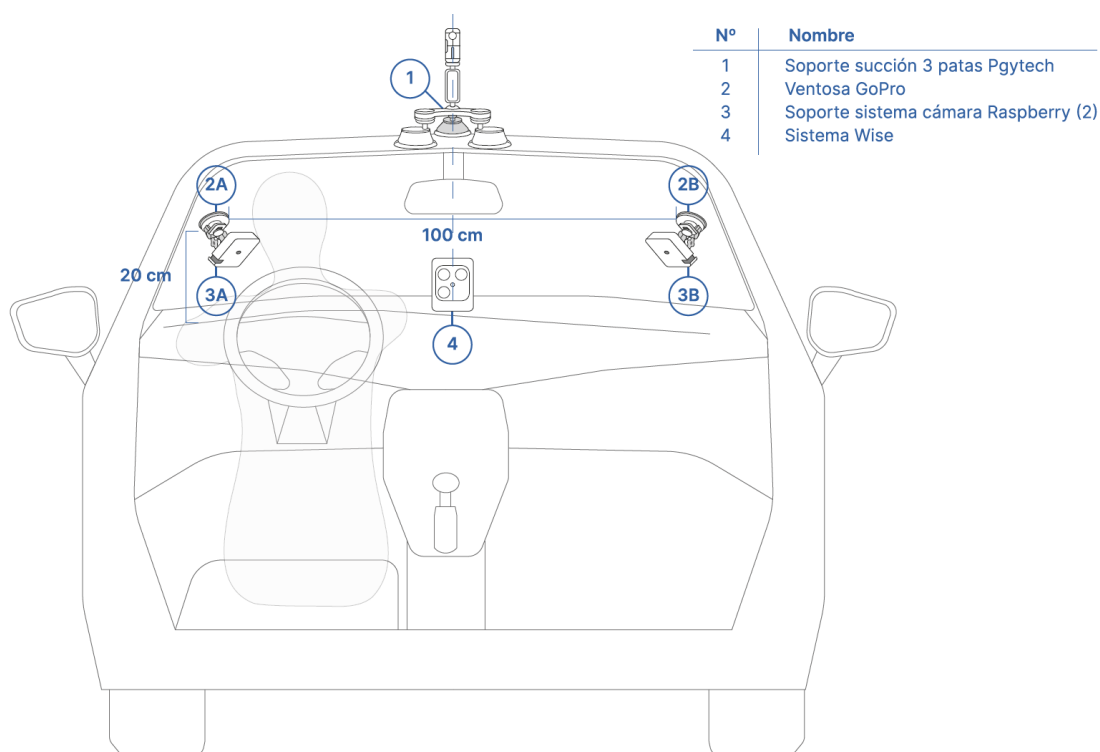
Figura 10: Plano de conjunto del montaje de los dispositivos de registro en el interior del vehículo.
