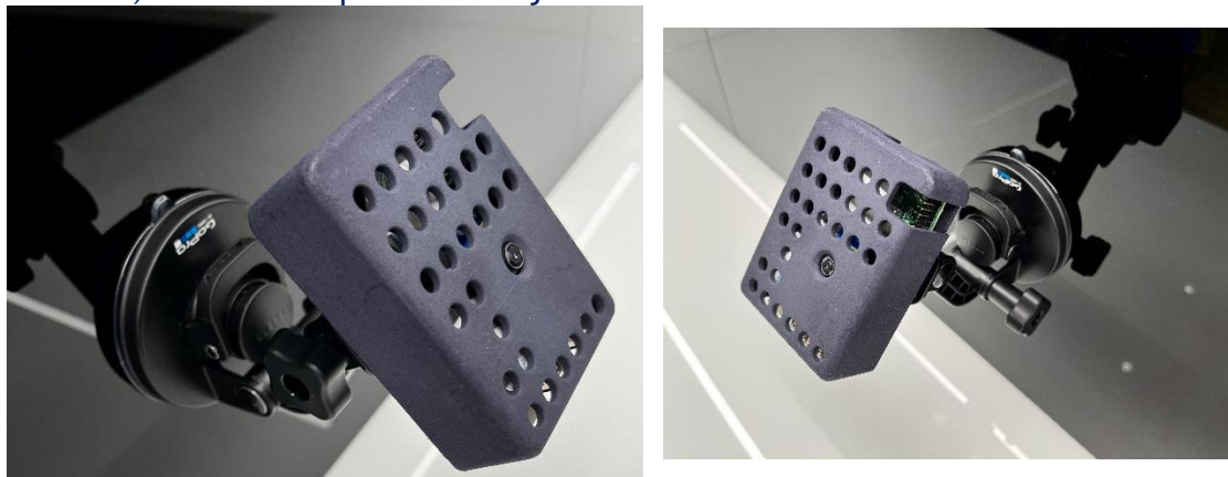
Figura 14: Imagen de los soportes de las cámaras montadas y fijadas mediante ventosa comercial.
