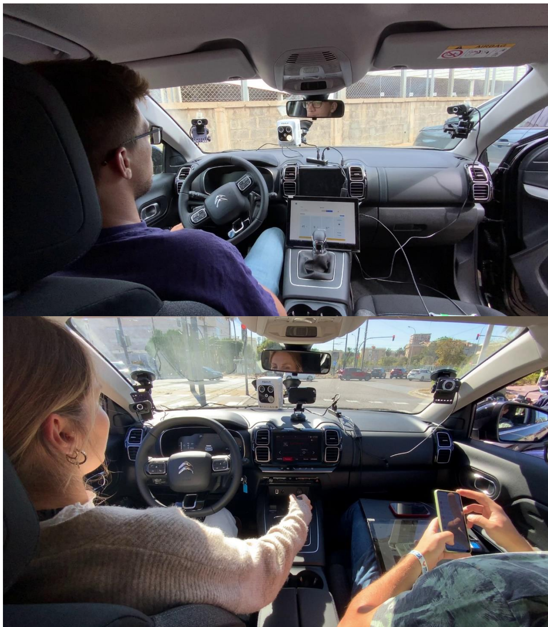
Figura 15: Imagen del sistema IBV iMoLab implementado en el vehículo.
