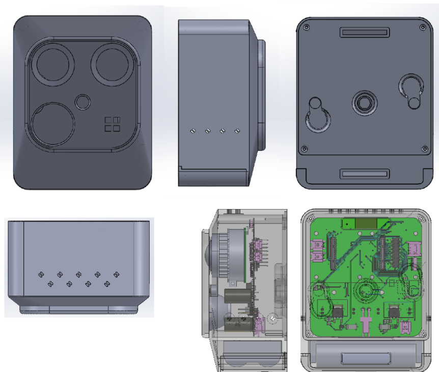
Figura 5: Sistema de registro no invasivo WISE
