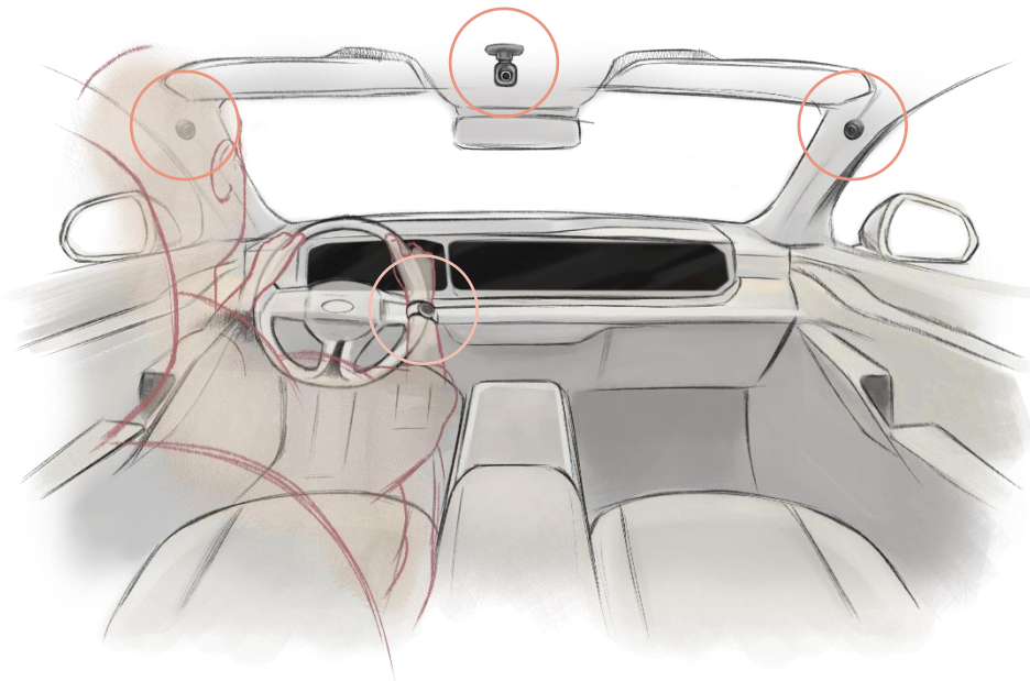
Figura 8: Boceto digital que muestra la ubicación de los diversos dispositivos del sistema
